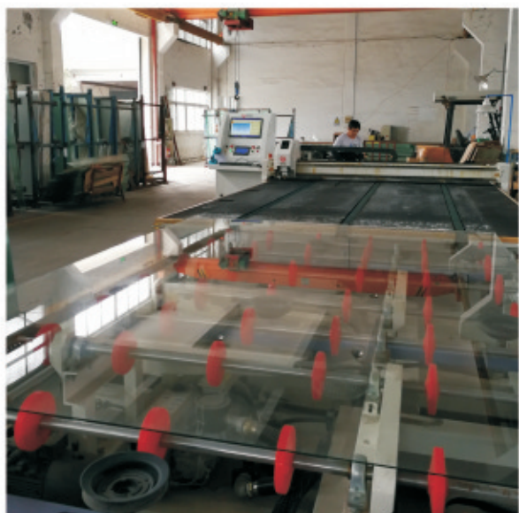
切割机 Cutting machine
